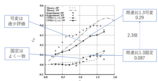
URANS結果と風洞実験結果の比較
