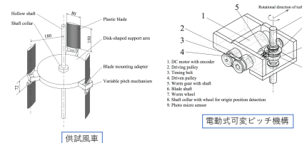
設計・製作した風洞実験用小型風車
