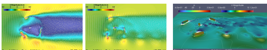
URANS解析例 (周速比1.3, 左: 固定, 右: 可変)
